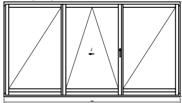
"C" villázat 1 bukó-toló szelvény, 2 nyíló szelvény
