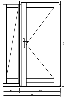
Egyszárnyú + fix oldalvilágító
