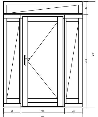
Egyszárnyú + 2 fix oldalvilágító + fix felülvilágító
