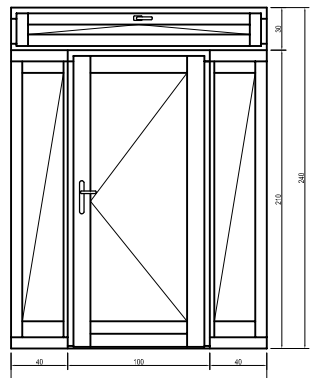
Egyszárnyú + 2 fix oldalvilágító + bukó felülvilágító
