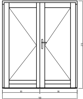
Kétszárnyú közepén felnyíló
