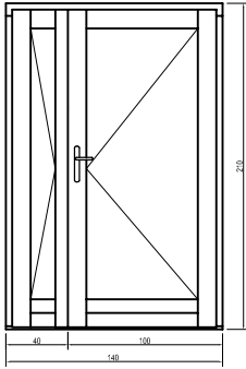
Kétszárnyú aszimmetrikusan felnyíló
