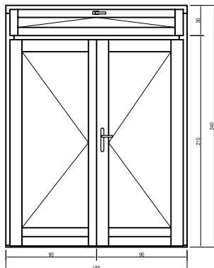
Kétszárnyú közepén felnyíló + bukó felülvilágító
