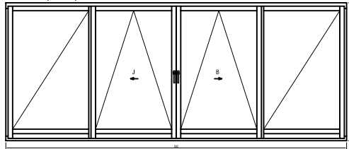
"C" villázat 2 bukó-toló szelvény, 2 nyíló szelvény
