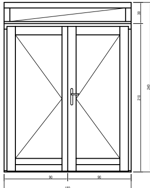
Kétszárnyú közepén felnyíló + fix felülvilágító
